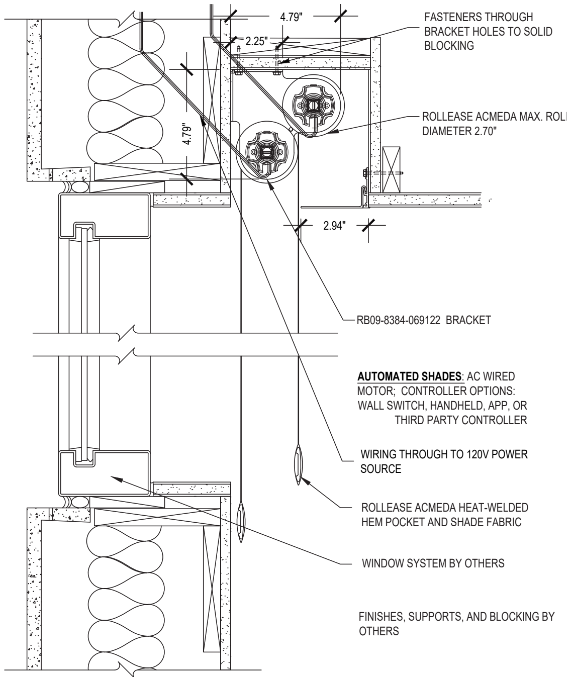
SCALE: 3"=1'-0" 120V AC MOTOR CONTROL
